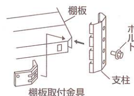
(図4) 棚板の取り付け方
