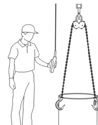
④バネの張力が無くなるまで下げて、フックをはずす。
